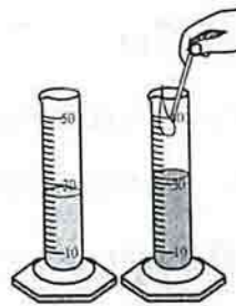
រូបទី ៥: ឱស្ទកម្មទឹកអុកស៊ីសែន កាតាលីសដោយអ៊ីយ៉ុង Fe^{3+} កែវក្រិតឆ្វែង : O_2 ភាយតិច (បរិមាណ Fe^{3+} តិចជាង) កែវក្រិតស្តាំ: O_2 ភាយច្រើន (បរិមាណ Fe^{3+} ច្រើនជាង)
