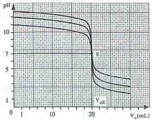
រូបទី ៨ : ខ្សែកោង \text{pH} = f(V_a) និងឥទ្ធិពលកំហាប់ ទៅលើការលោត \text{pH}
