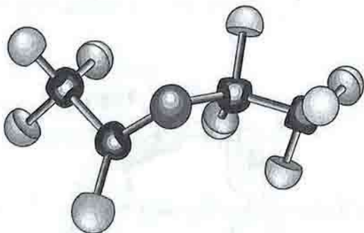
រូបទី ៤ : គំរូម៉ូលេគុលនៃអេស៊ីលអេតាណូអាត រឺអេស៊ីលអាសេតាត CH_3-COOC_2H_5
