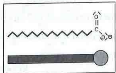
រូបទី ៤ : គំនូសតាងអ៊ីយ៉ុងកាបូកស៊ីឡាតនៃសាប៊ូ
