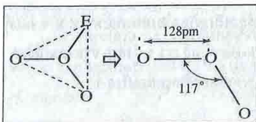
រូបទី ១៩ : ម៉ូលេគុលអូសូន \text{O}_3 ជាបង្អែង
