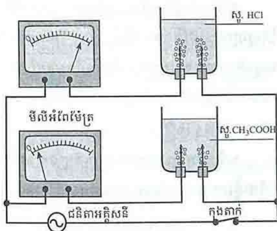
រូបទី ២: សូលុយស្យុងអាស៊ីតអេតាណូអ៊ីចចំលងចរន្ត ខ្សោយជាងសូលុយស្យុងHCl
