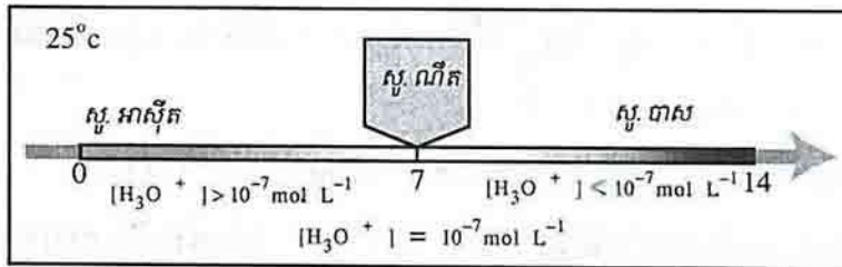
រូបទី៦ : សូលុយស្យុងអាស៊ីត បាស និងណឺត : pH និង [H_3O^+] នៅ 25^{\circ}C
