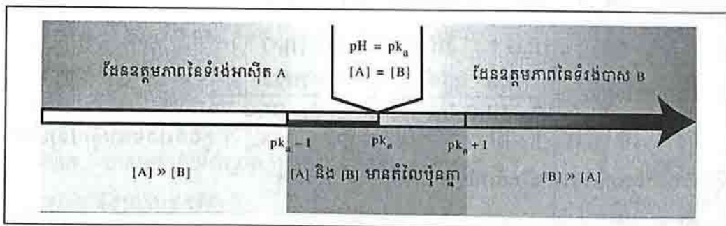
រូបទី ១: ដែនឧត្តមភាពនៃទំរង់ឆ្លាស់ទាំងពីរបស់កូ A/B
