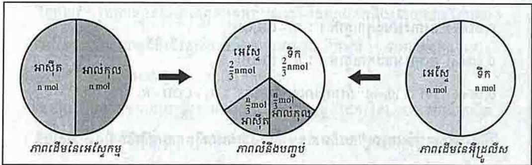
រូបទី ១០ : គេទទួលបានភាពលំនឹងដូចគ្នាដោយដោយផ្ដើមពីល្បាយស្មើម៉ូលនៃអាស៊ីត និងអាល់កុល រឺ អេស្តែ និងទឹក
