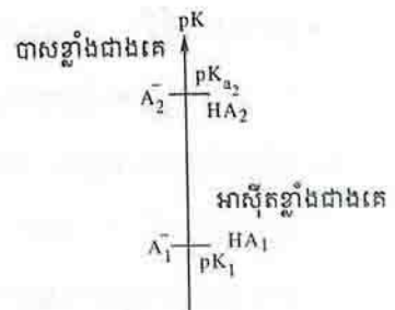
រូបទី៣: ទិសដៅប្រតិកម្មអាស៊ីតបាសរវាងពីរគូអាស៊ីត - បាស
