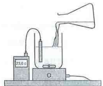
រូបទី ១ : ប្រតិកម្មរវាង HCl និង NaOH បញ្ចេញកំដៅ
