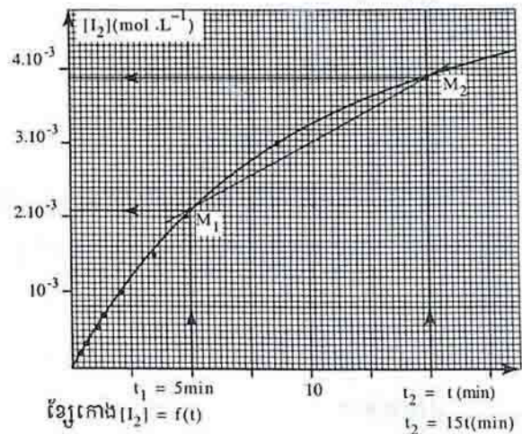
ល្បឿនមធ្យមនៃកំហាប់ I_2 ចន្លោះពេល t_1 និង t_2 ស្មើនឹងមេគុណប្រាប់ទិសនៃបន្ទាត់ M_1M_2
