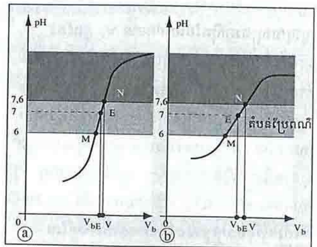
រូបទី ១១: ឥទ្ធិពលនៃកំហាប់សូលុយស្យុងលើភាពជាក់លាក់នៃអត្រាអាស៊ីតខ្លាំង-បាសខ្លាំងនៅចំពោះមុខប្រូម៉ូទីម៉ុលខៀវ
