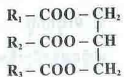
រូបទី ២ : រូបមន្តស្ទើរលាតនៃទ្រីគីសេរីត
