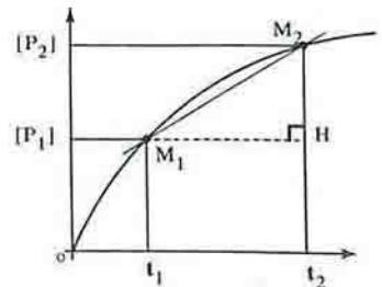
កំនត់តាមក្រាហ្វិចនូវល្បឿនមធ្យមនៃកំនត់អង្គធាតុកើត P នៅចន្លោះ t_1 និង t_2
