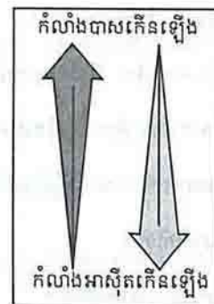
រូបទី ២ : កំលាំងអាស៊ីតរឺបាសនៃតួមួយជាអនុគមន៍នៃ K_a រឺ pK_a
