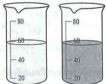
រូបទី ៩: ឥទ្ធិពលជាកាតាលីករនៃ Mn^{2+} ទៅលើអេដុកម្ម MnO_4^- ដោយអាស៊ីតអុកសាលិច បេស៊ីឆ្នេងដែលមានអ៊ីយ៉ុង បំរែពណ៌នៃ ល្បឿនជាង ។
