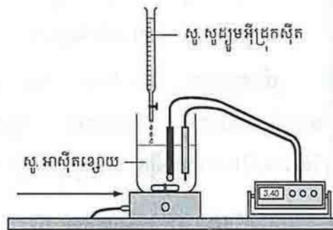
រូបទី៧: អត្រា pH មេទ្រីចនៃសូលុយស្យុងអាស៊ីតខ្សោយ ដោយសូលុយស្យុង NaOH
