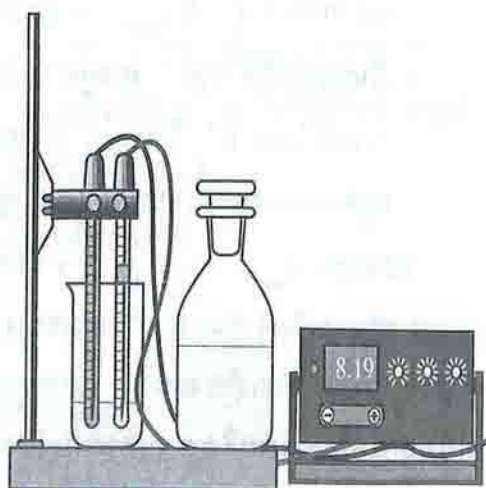
រូបទី ៥ : វាស់ pH នៃសូលុយស្យុងសូដ្យូមអេតាណូអាត ទើបរៀបចំថ្មីៗ
