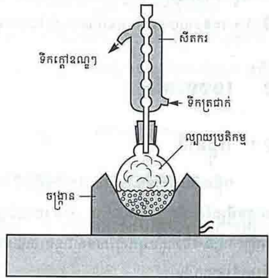
រូបទី ១ : ទង្វើអេស្ទែដោយដាក់កំដៅល្បាយអាស៊ីត និងអាល់កុលជាមួយកាតាលីករ
