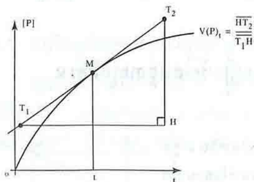
កំនត់តាមក្រាហ្វិច : ល្បឿនកំនើតអង្គធាតុកើត P នៅខណៈពេល t
