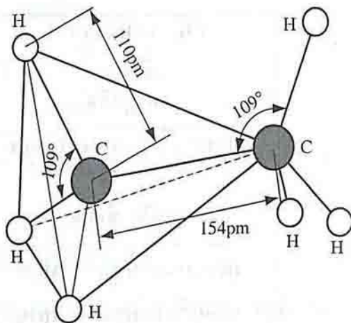
រូបទី ១២ : ម៉ូលេគុលអេតានមានអាតូមកាបូនចតុមុខ 2 ។
