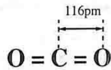
រូបទី១៦ : គំរូម៉ូលេគុល \text{CO}_2
