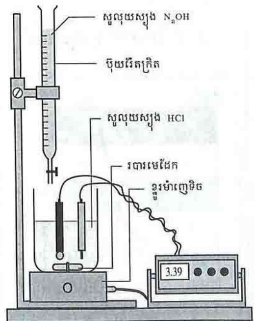
រូបទី ៩ : ដំនើរការពិសោធន៍នៃអត្រា pH មេទ្រីចនៃ សូលុយស្យុងអាស៊ីតដោយសូលុយស្យុងធាន
