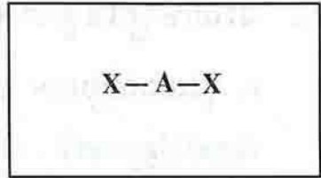
រូបទី ១១ : ទំរង់ទ្រូងក្រុងប្រភេទ \text{AX}_2
