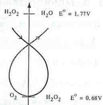
រូបទី៣: តួអ្នកទាំងពីរនៃទឹកអុកស៊ីសែន និងវិធានការ
