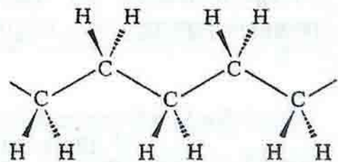
រូបទី ១៥ : ទ្រង់ទ្រាយបង្អិតបានធ្វើអោយខ្សែកាបូន មានភាពជាបន្ទាត់ក្លិចកូក
