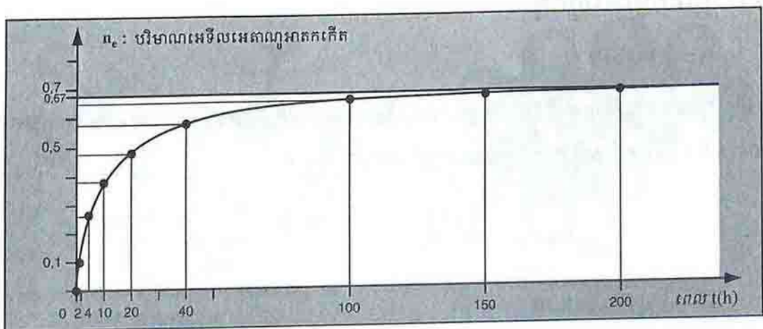
រូបទី 7 : ខ្សែកោងបង្ហាញពីបំរែបំរួលបរិមាណអេស្ត្រអេតាណូអ៊ីតដែលកើតជាអនុគមន៍នឹងរយៈពេល : n_e = f(t)
