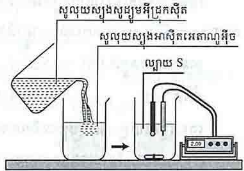
រូបទី ៣: ទង្វើនិងរាង pH នៃសូលុយស្យុងនៅពាក់កណ្តាលសមមូលនៃប្រតិកម្មអាស៊ីតអេតាណូអ៊ីច និងស្ទូត ។
