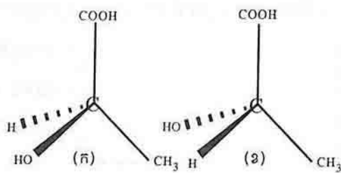
រូបទី 9 : រូបសណ្ឋាន 2 នៃអាស៊ីត 2-អ៊ីដ្រូកស៊ីប្រូប៉ាណូអ៊ិច
