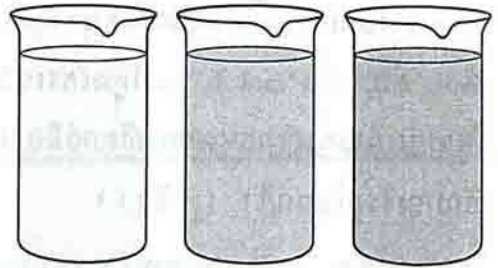
រូបទី 2 : ឥទ្ធិពលនៃកំហាប់ H_2O_2 ទៅលើស៊ីនេទិចនៃអេកមូរបស់វាដោយអ៊ីយ៉ុង I^- ពណ៌នៃសូលុយស្យុងកាន់តែជឿងពីបេស៊ែទី 1 (ខាងឆ្វេង) ទៅបេស៊ែទី 2 (ខាងស្តាំ)
