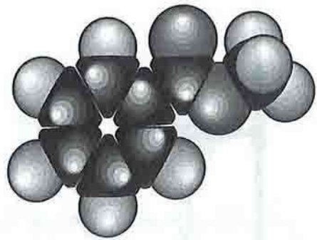
រូបទី ៥ : គំរូម៉ូលេគុលនៃមេស៊ីលបង់សូអាត C_6H_5-COOCH_2CH_3
