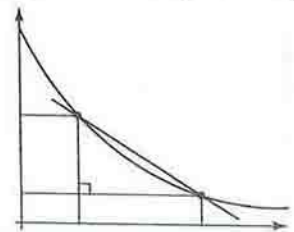
កំនត់តាមក្រាហ្វិចនូវល្បឿនមធ្យមនៃបំបាត់វិវេណកំទីប R ចន្លោះពេល t_1 និង t_2
