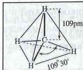
រូបទី ២០ : ធរណីមាត្រតេត្រាអ៊ែតនៃ \text{CH}_4
