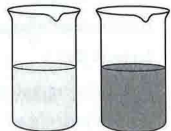
រូបទី ១: ឥទ្ធិពលនៃកាតាលីករអាម៉ូញ៉ូមម៉ូលីបដាតទៅលើអុកស៊ីតកម្មនៃអ៊ុយរ៉ង់ I^- ដោយ H_2O_2 កែវបេស៊ីស្តាំមានកាតាលីករ កំន I_2 លឿន ។
