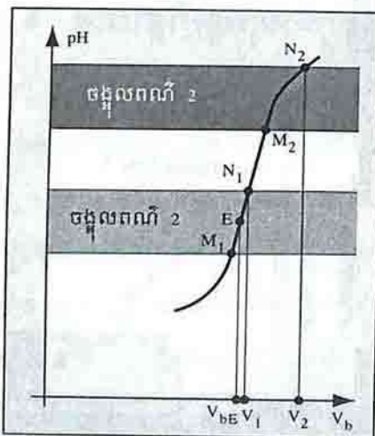
រូបទី ១០: ជំរើសអង្គធាតុចង្អុលពណ៌
