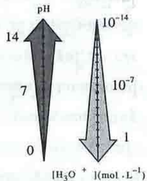
រូបទី ៤ : pH និងកំហាប់ [H_3O^+] ប្រែប្រួលក្នុងទិសដៅផ្ទុយគ្នា
