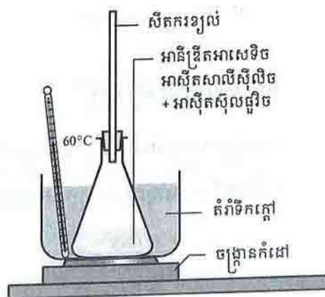
រូបទី ២ : ឧបករណ៍ទង្វើអាស្ត័រិន
