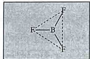
រូបទី 17 : ធរណីមាត្រត្រីកោណនៃ \text{BF}_3
