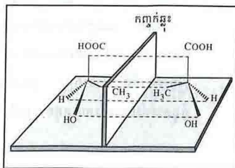
រូបទី 10 : រូបឆ្លុះគ្នានៃរូបសណ្ឋានទាំងពីរនៃអាស៊ីត 2-អ៊ីដ្រូកស៊ីប្រូប៉ាណូអ៊ិច
