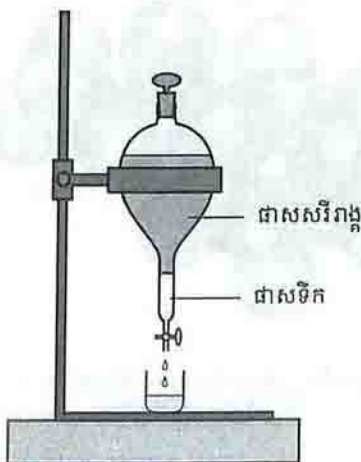
រូបទី ២ : យោបកជាសទឹកដោយធាតុរំលាយសរីរាង្គក្នុងអំពូលច្រោះ
