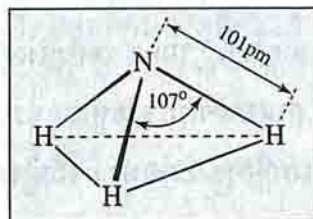
រូបទី ២២ : ធរណីមាត្រពីរ៉ាមីតនៃម៉ូលេគុល NH_3
