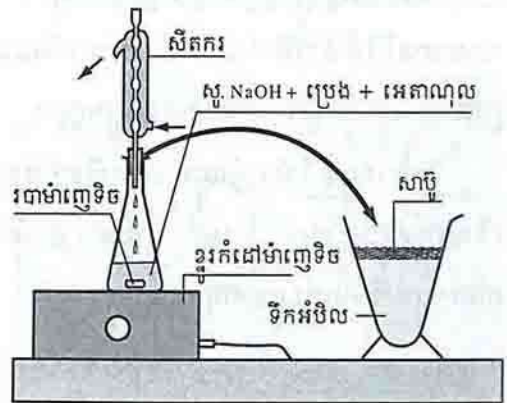
រូបទី ៣ : ទង្វើសាប៊ូដោយសាប៊ូកម្មប្រេង
