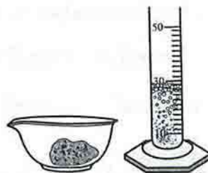
រូបទី ៦: កាតាលីសដោយអង់ស៊ីមនៃឱស្ទកម្មទឹកអុកស៊ីសែន ប្រើកាតាឡាសនៃឈាម ។
