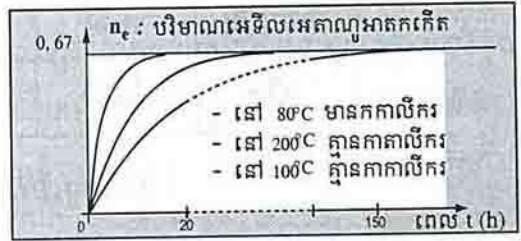
រូបទី ៨ : ឥទ្ធិពលនៃសីតុណ្ហភាព និងកកាសិករលើការវិវត្តនៃ បរិមាណអេស្បែកដែលកើតឡើងដោយល្បាយស្មើមួយនៃ អាស៊ីតអេតាណូអ៊ីច និងអេតាណុល
