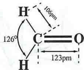
រូបទី 18 : គំរូម៉ូលេគុលនៃ \text{CH}_2\text{O}
