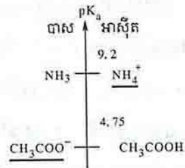
រូបទី ៦ : ប្រតិកម្មនៃអ៊ីយ៉ុងអាម៉ូញ្យូមជាមួយអ៊ីយ៉ុងអេតាណូអាតជាប្រតិកម្មកំរិតបំផុត
