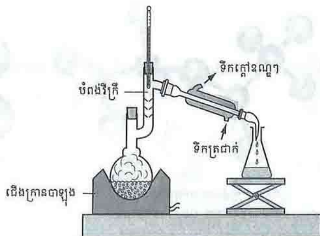
រូបទី ៣ : បំនិតដើម្បីញែកធាតុបង្កនៃល្បាយ
