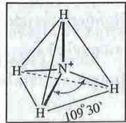
រូបទី ២១ : ធរណីមាត្រនៃអ៊ីយ៉ុង \text{NH}_4^+
