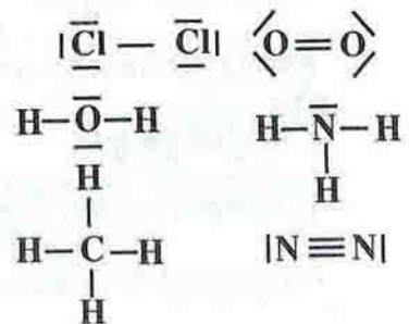
រូបទី៣ : ឧទាហរណ៍បង្ហាញពីវិធានអដ្ឋតា
