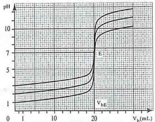
រូបទី ៧ : ឥទ្ធិពលនៃកំហាប់សូលុយស្យុងទៅលើការលោត \text{pH}
