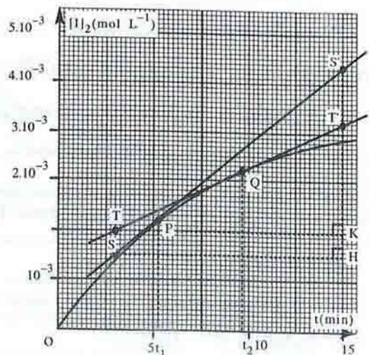
រូបទី 3 : ល្បឿននៃ I_2 ថយតាមពេល ។ តាមការគណនាមេគុណប្រាប់ទិសត្រង់ Q និង P នៃខ្សែកោង [I_2] = f(t) គេដឹងថា V(I_2)_{t_2} តូចជាង V(I_2)_{t_1}
